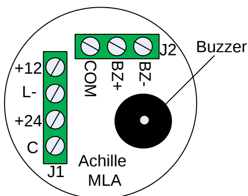
Connettore a vite/ Screw connector
