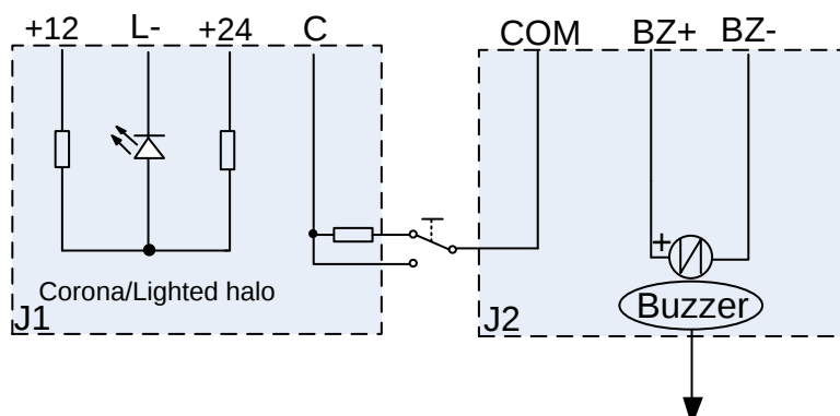
Schema di collegamento/ wiring diagram
